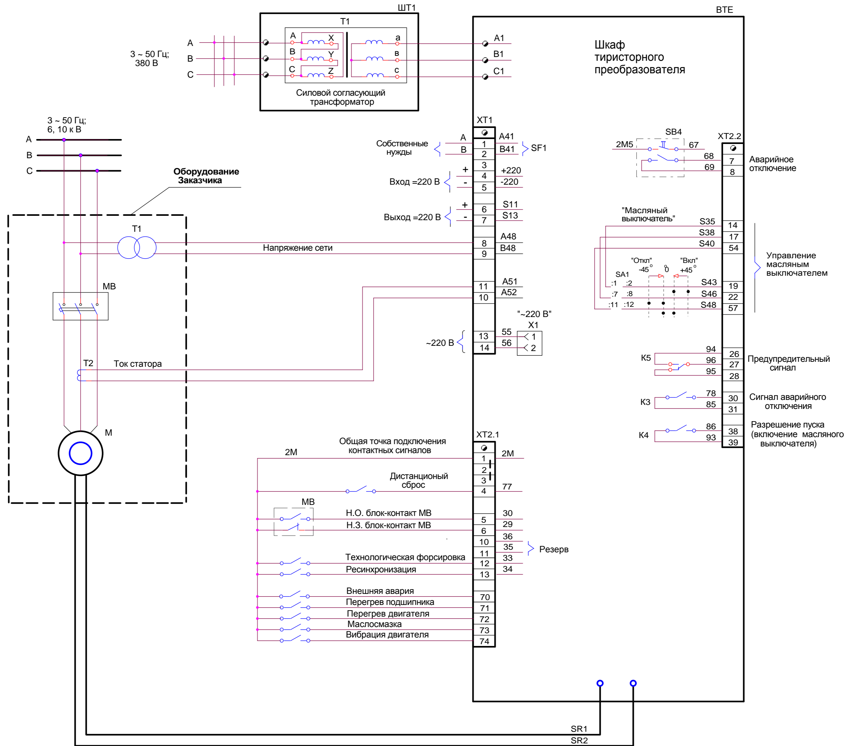
Схема с минимальным количеством подключений: прямой пуск
