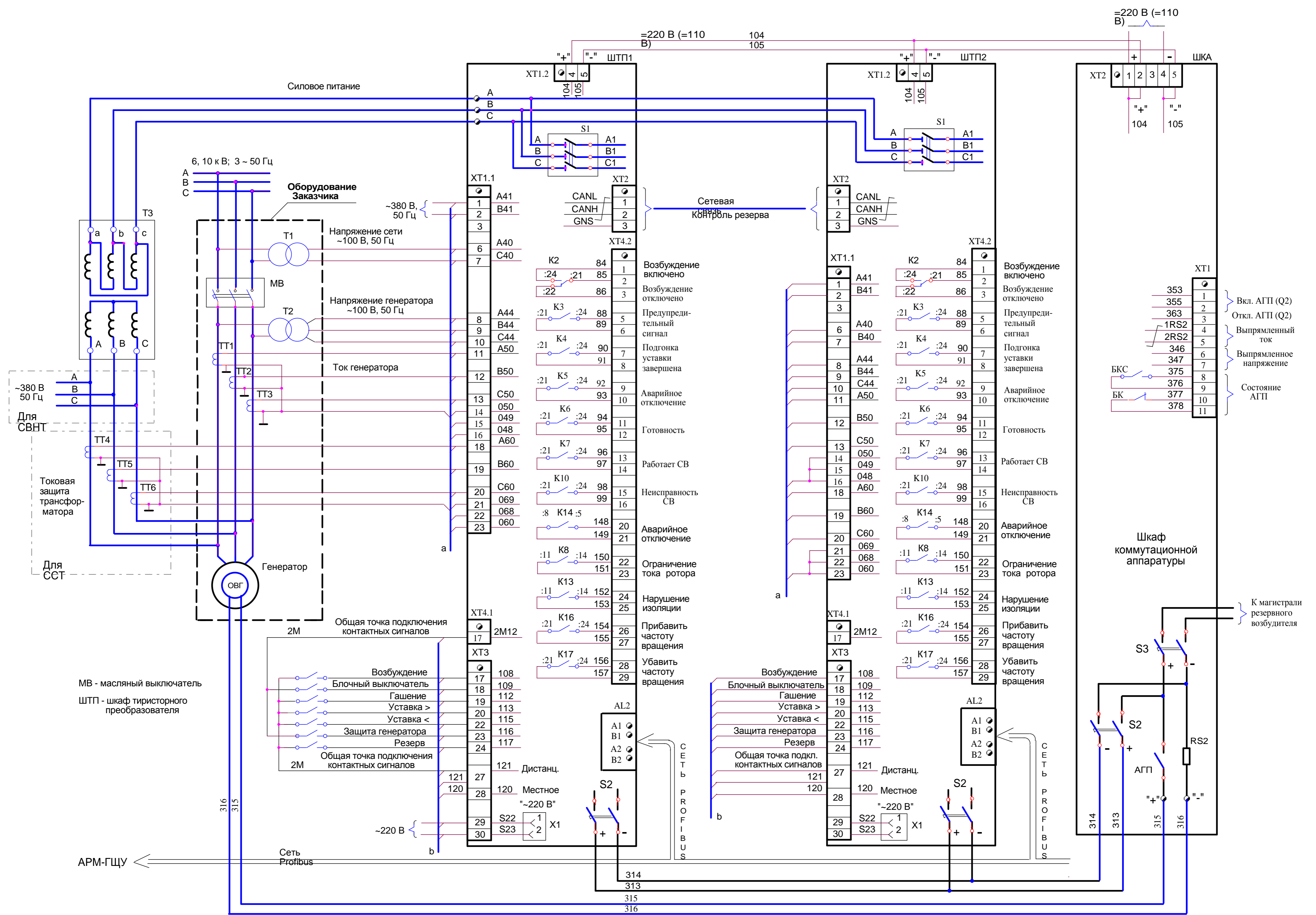
СВНТ/ССТ: Схема с максимальным количеством подключений: автосинхронизация, контроль 3-х фаз тока и напряжения, АГП, КСС, горячий резерв, внешнее резервное возбуждение, сетевая связь
