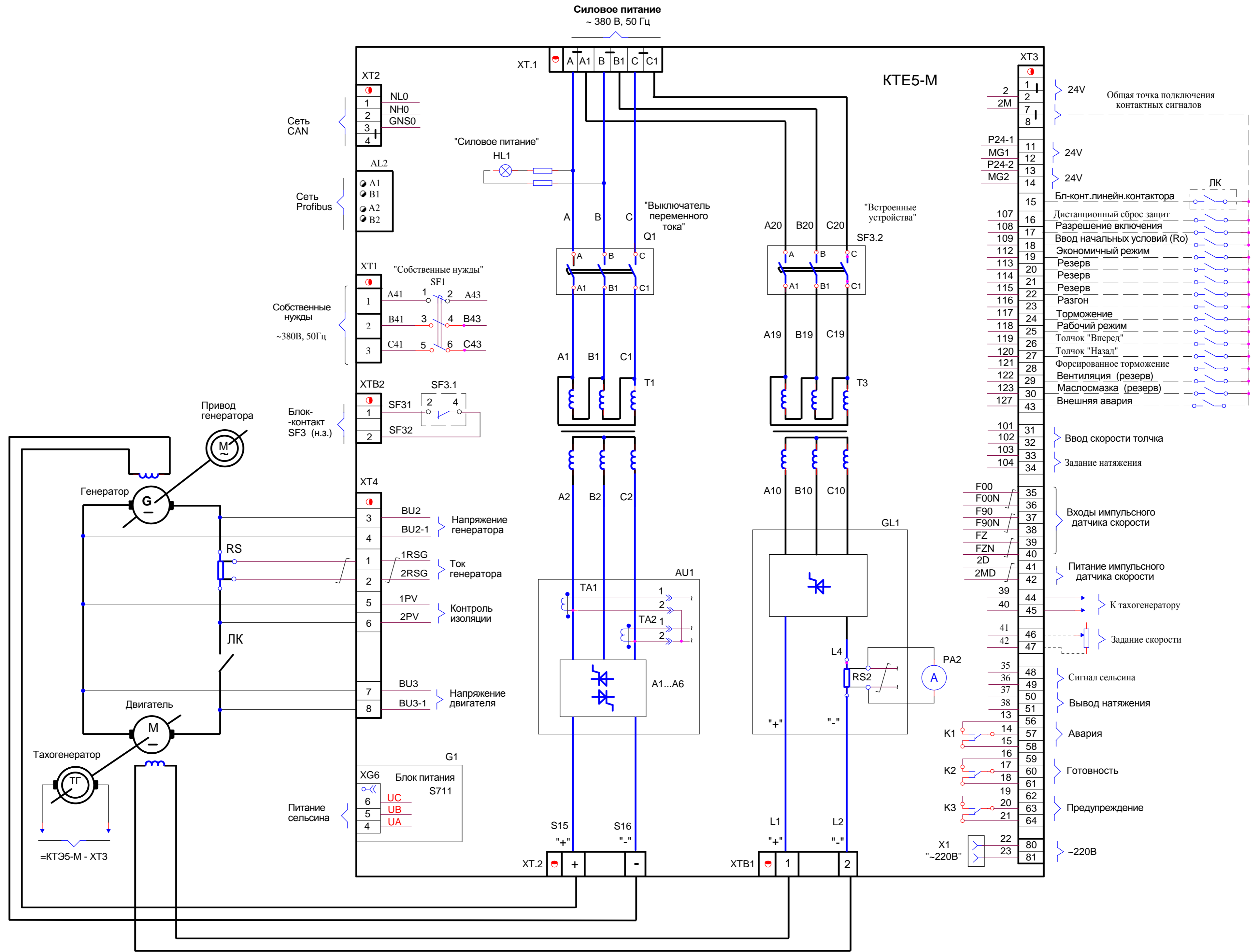
Электропривод моталки. Система генератор-двигатель. Схема подключений
