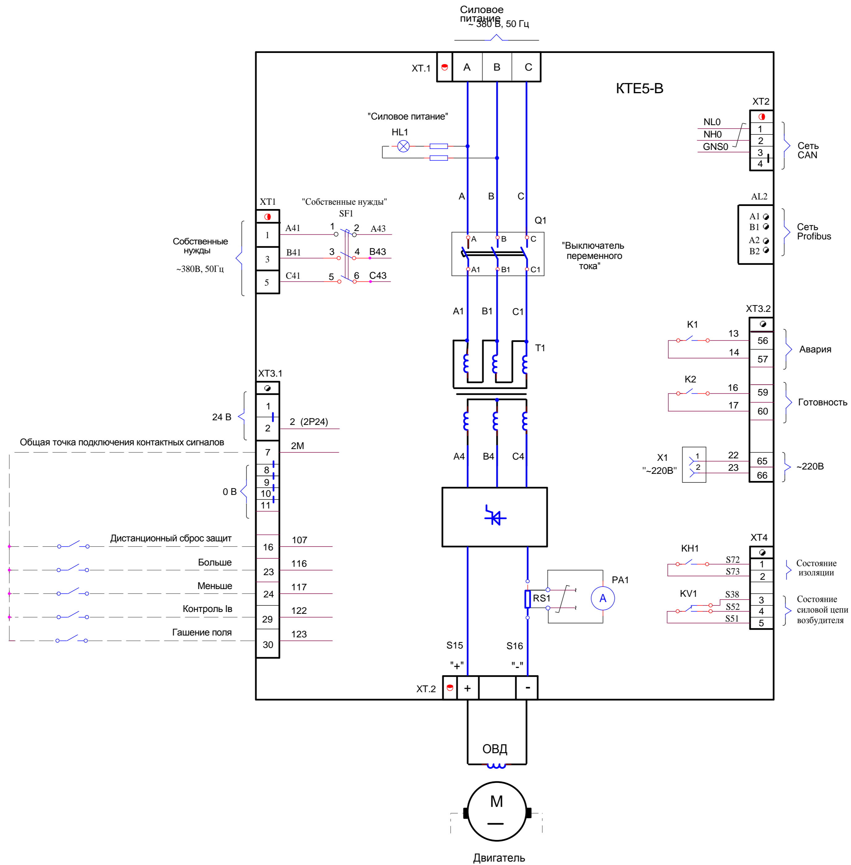
Возбудитель привода постоянного тока. Схема подключений
