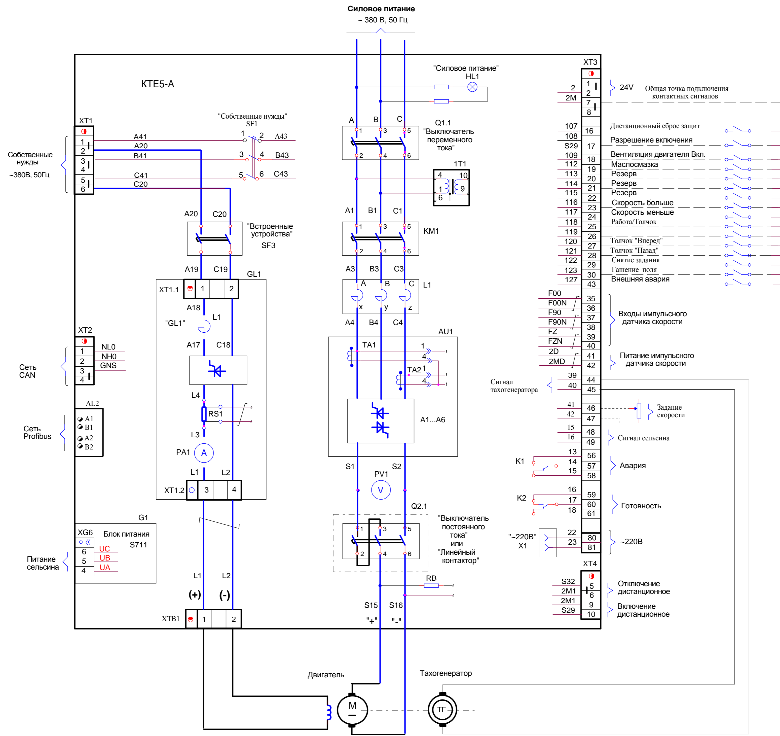
Электропривод базового исполнения. Схема подключений
